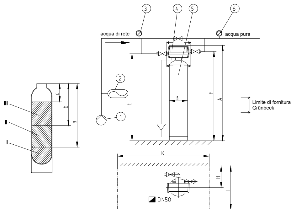
Fig. 2: disegno di installazione con disegno di fondazione
