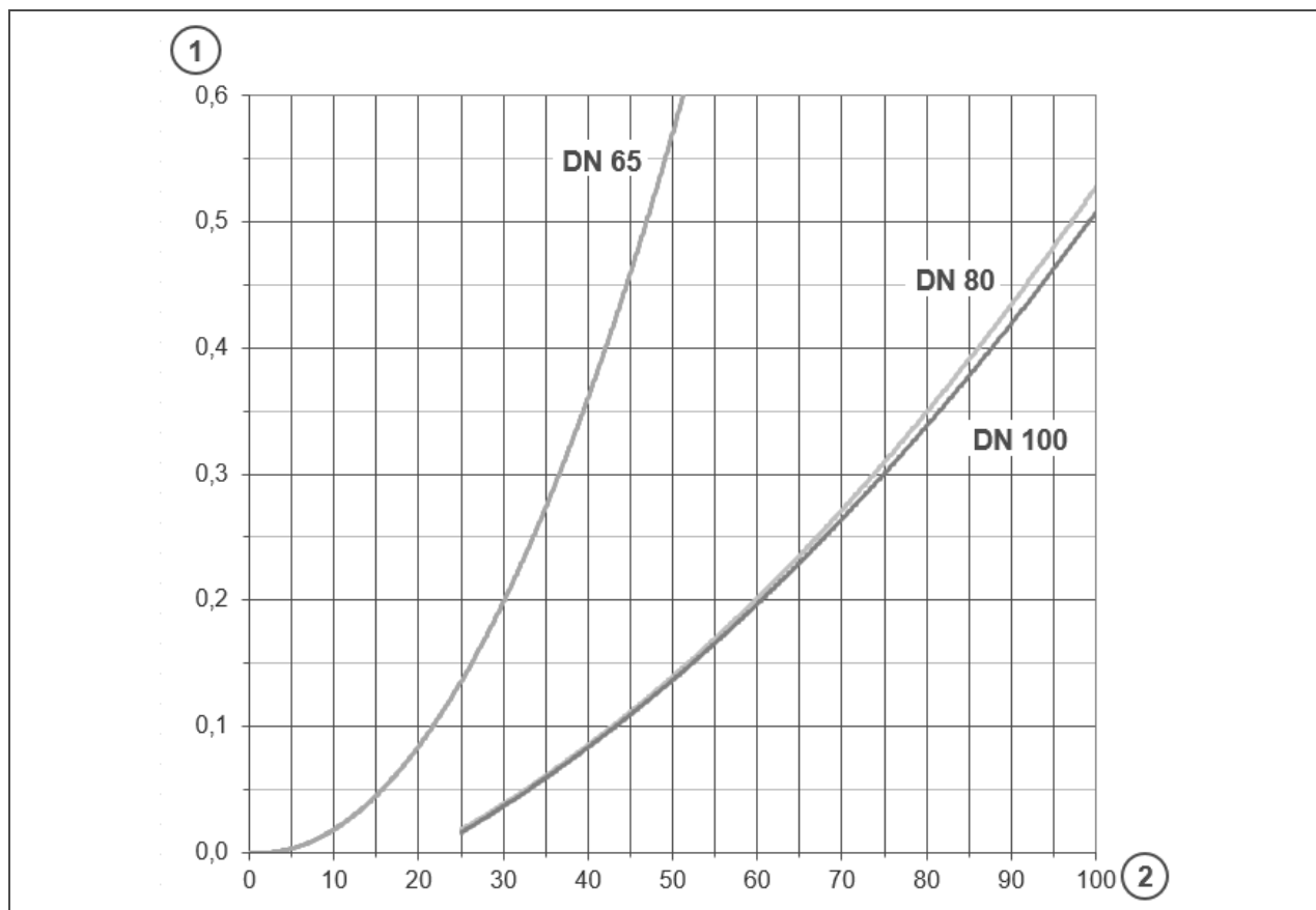
Druckverlustkurven Rückspülfilter MR65/MR80/MR100
