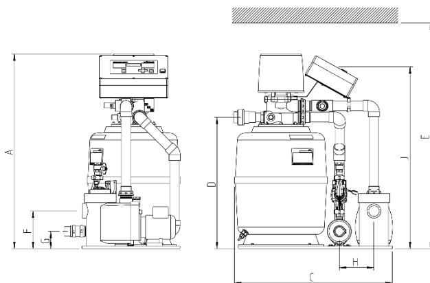
Abb. 2 Maßzeichnung Filteranlage GENO-mat F 500 AK
