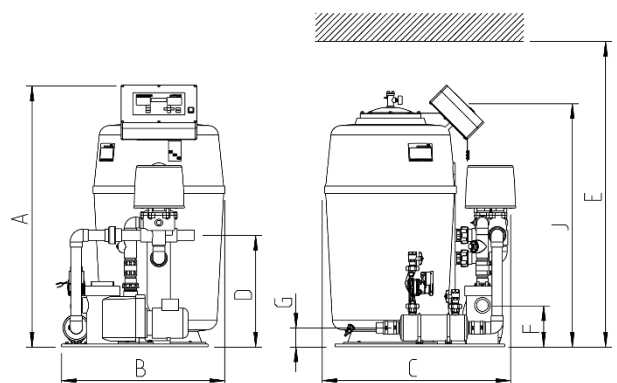
Abb. 3 Maßzeichnung Filteranlage GENO-mat F 600 AK
